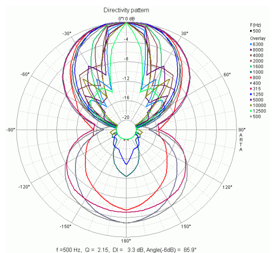
Polardiagramm
