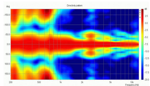
Isobarendiagramm
